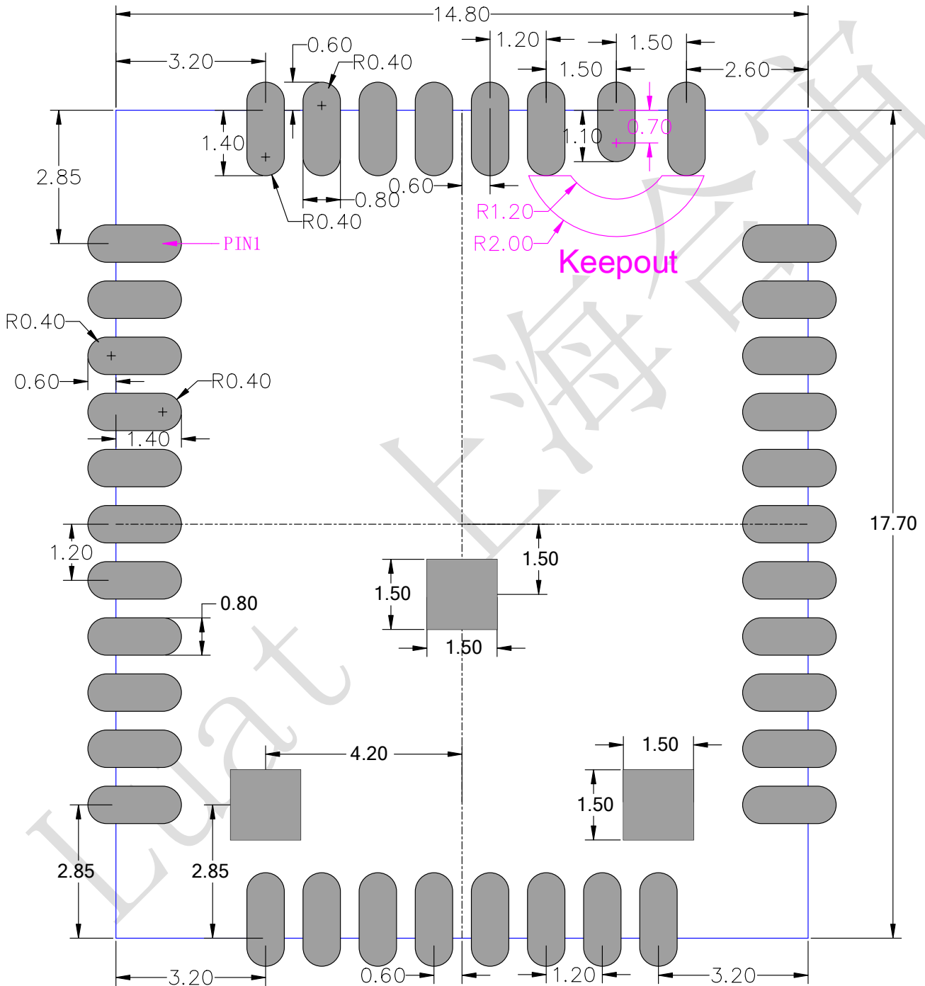
图表 29: 推荐封装 (单位: 毫米)
