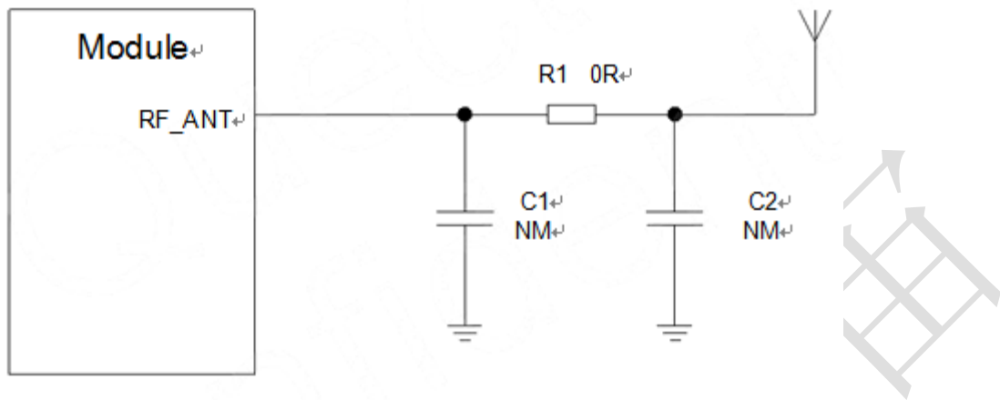
图表 26: 射频参考电路
