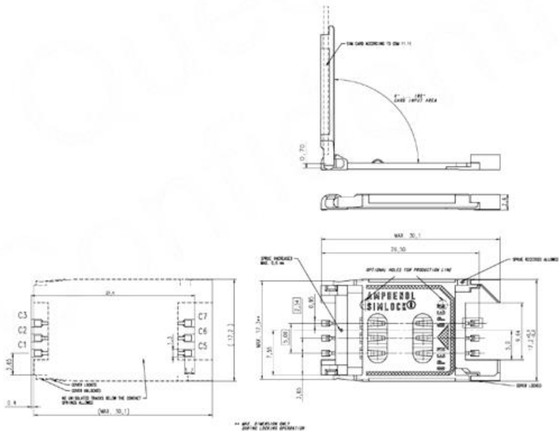
图表 20: Amphenol C707 10M006 512 2 SIM 卡座
